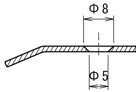
断面 A-A
